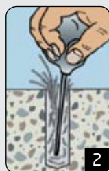
2 Почистить отверстие
