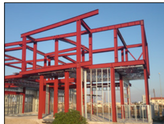
Крепление металлических конструкций.
